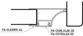
Rysunek techniczny produktu | product technical drawing | технический чертеж
