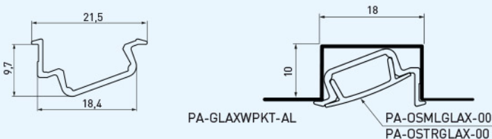
Rysunek techniczny produktu | product technical drawing | технический чертеж
