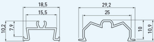
Rysunek techniczny produktu | product technical drawing | технический чертеж
