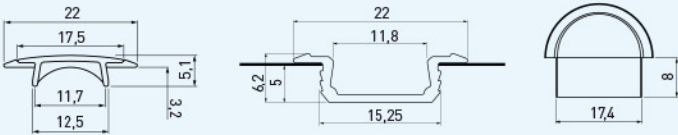
Rysunek techniczny produktu | product technical drawing | технический чертеж
