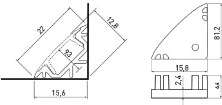
Rysunek techniczny produktu | product technical drawing | технический чертеж
